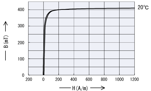
Static Magnetization Curves 直流比行リシ特性
