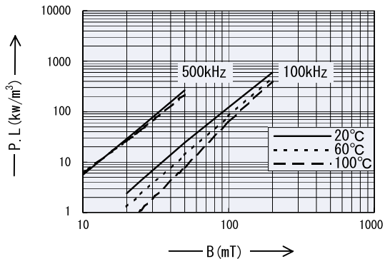
Power loss vs. Flux density P^{\circ} ワロス vs. 磁束密度
