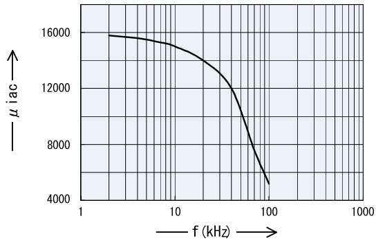
\mu_{iac} vs. Frequency \mu_{iac} 周波数特性
