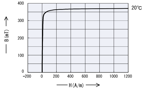
Static Magnetization Curves 直流比励磁特性
