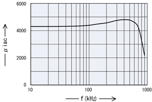
\mu_{iac} vs. Frequency \mu_{iac} 周波数特性
