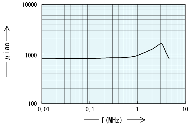
\mu_{iac} vs. Frequency \mu_{iac} 周波数特性
