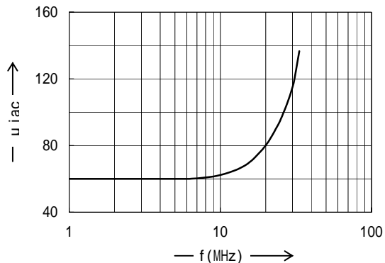
\mu_{iac} vs. Frequency \mu_{iac} 周波数特性
